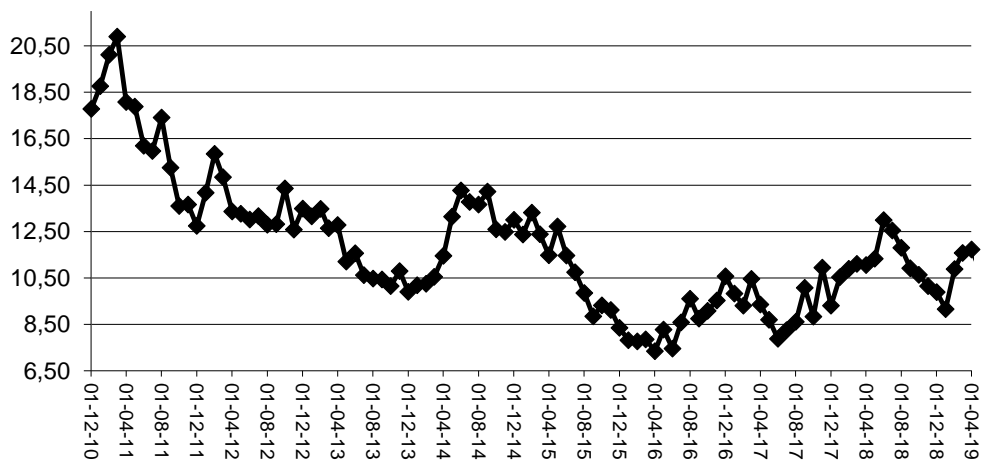
Ni (€/kg) 2010 - 2019
