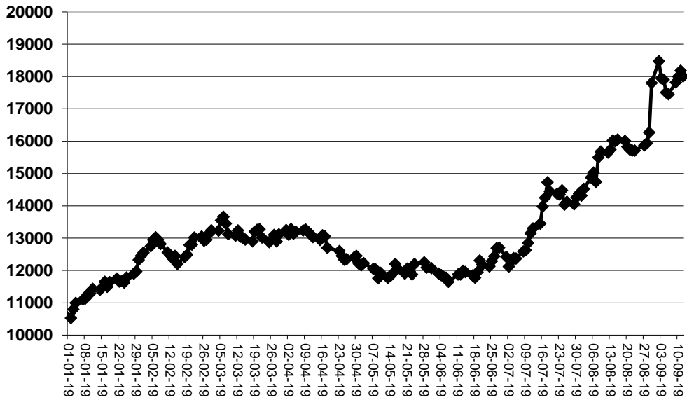
Ni ($/To) 2019
